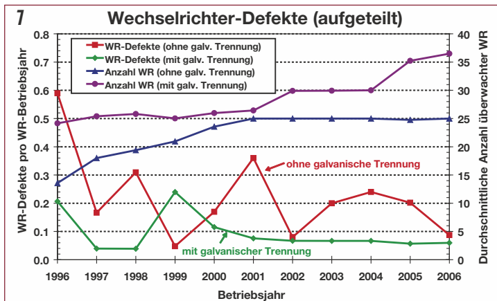
Bild 7 Wechselrichter-Defekte pro Wechselrichter-Betriebsjahr aufgeteilt nach Geräten mit und ohne galvanische Trennung. Die Wechselrichter ohne galvanische Trennung haben tendenziell eine höhere Ausfallrate. Allerdings stammen praktisch alle überwachten Wechselrichter ohne galvanische Trennung vom gleichen Hersteller. Deshalb ist diese Betrachtung nur bedingt repräsentativ.
