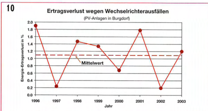
Bild 10 Energie-Ertragsverluste in Prozent auf Grund von Wechselrichter-Defekten bei den überwachten Anlagen. Der Mittelwert liegt bei 1,1%.
