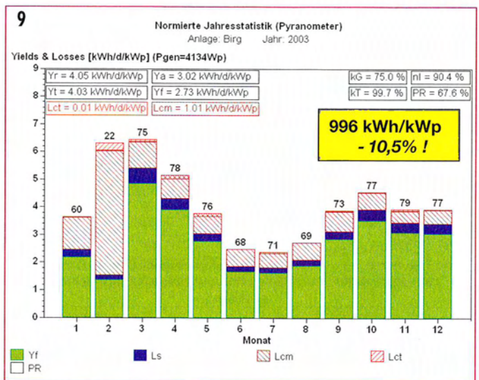
Bild 9 Normierte Jahresstatistik für 2003 der Anlage Birg (2670 m). Im Jan./Feb. trat ein schwerwiegender Wechselrichter-ausfall auf, der einen Ersatz des Gerätes erforderlich machte. Energieverlust: -10,5%.
