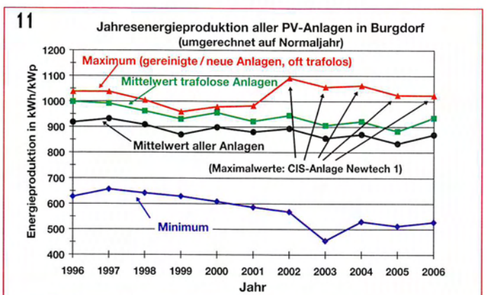
Bild 11 Spezifische Jahresenergieproduktion aller PV-Anlagen mit Wechselrichtern in Burgdorf in den Jahren 1996–2006 (bezogen auf die vom Hersteller deklarierte Solar-generator-Nennleistung). Der Anstieg des Maximums ab 2002 ist auf die neu in Betrieb genommene Dünnschichtzellen-Anlage Newtech 1 [1], [4], [5] zurückzuführen.
