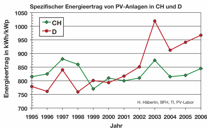
Bild 2 Mittlerer spezifischer Energieertrag netzgekoppelter PV-Anlagen in den Jahren 1995 – 2006 in Deutschland und der Schweiz. In den ersten Jahren ist der CH-Ertrag entsprechend den besseren Strahlungsverhältnissen etwas grösser (Grafik aus [1], aufdatiert mit neuesten Werten für 2006 aus den gleichen Datenquellen).
