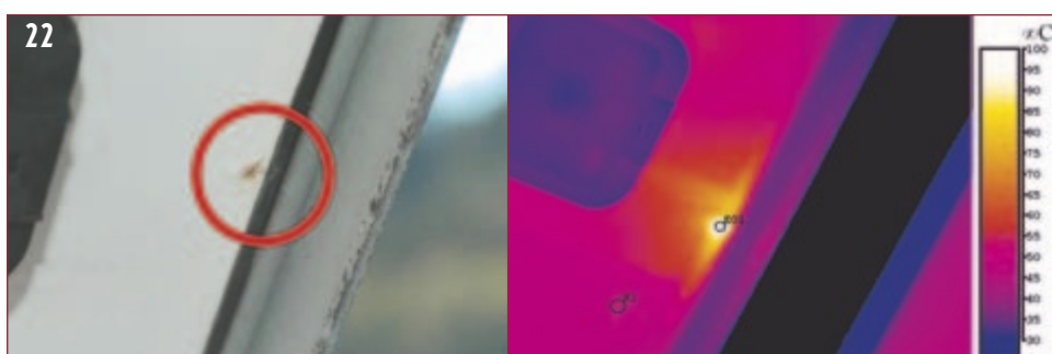
Bild 22 Auf der Rückseite ist auch die Folie durchgeschmolzen. Die Stelle erwärmt sich massiv (> 86°C!). Bei manchen älteren Anlagen sind auf thermografischen Aufnahmen des Solargenerators elfliche solche heisse Stellen zu finden, die längerfristig zu Schäden führen dürften.
