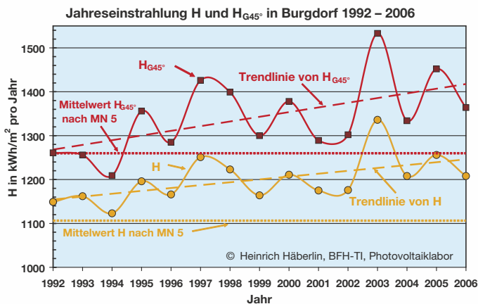
Bild 1 Jahreswerte der Einstrahlung H in die Horizontalebene und der Einstrahlung H_{G45^\circ} in eine um 45^\circ geneigte, genau südorientierte Ebene bei der zentralen Meteo-Messstation der BFH in Burgdorf in den Jahren 1992–2006. Zudem sind auch noch die Mittelwerte von H und H_{G45^\circ} gemäss dem Programm Meteororm 5 angegeben, das die Berechnung der Einstrahlung in beliebig orientierte Flächen ermöglicht [1].
