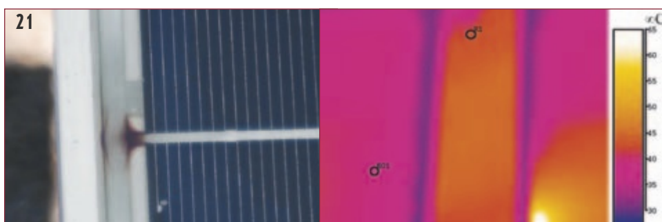
Bild 21 Stark erhitzter Kontaktstreifenübergang: Bei diesem Modul ist schon optisch feststellbar, dass der Übergangswiderstand der Kontaktstreifen zu gross ist und sich die Stelle stark erwärmt.
