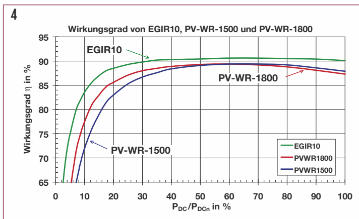
Bild 4 Umwandlungs-Wirkungsgrad \eta von Wechselrichtern (mit Trafo) um 1990 [1].
