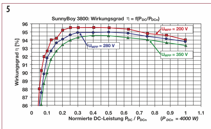
Bild 5 Umwandlungs-Wirkungsgrad \eta eines modernen Wechselrichters mit galvanischer Trennung. Der Wirkungsgrad ist nicht nur von der Leistung, sondern auch von der DC-Spannung abhängig [1]. Traflose Geräte erreichen noch etwa 2% höhere Werte.
