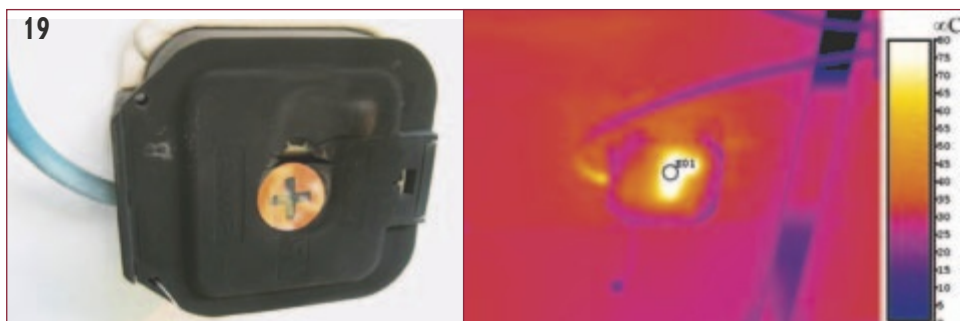
Bild 19 Geschmolzene Anschlussdose: Schon bei geschlossener Anschlussdose konnte am Punkt E01 (siehe thermografische Aufnahme rechts) eine Temperatur von über 80°C gemessen werden. Der Deckel ist durchgeschmolzen.
