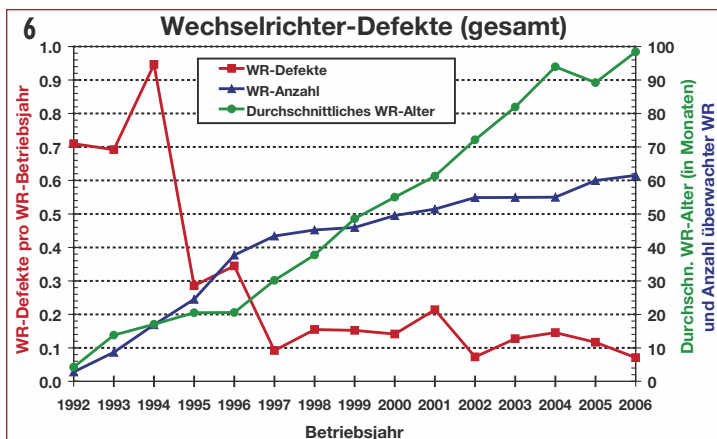
Bild 6 Wechselrichter-Defekte pro Wechselrichter-Betriebsjahr und durchschnittliche Anzahl vom PV-Labor der BFH in Burgdorf überwachter Wechselrichter. Die Ausfallrate hat im Jahr 2006 mit 0,07 Defekten pro WR-Betriebsjahr erneut einen Rekordtiefstand erreicht. Die Anzahl überwachter WR ist immer noch am Steigen (Ende 2006: 61 Geräte). Das durchschnittliche Alter der Wechselrichter beträgt etwa 8 Jahre.
