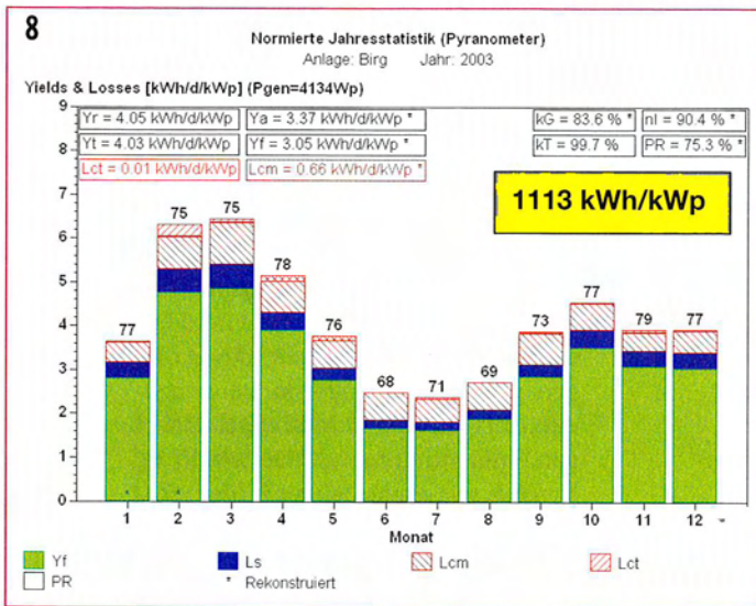
Bild 8 Normierte Jahresstatistik für 2003 der Anlage Birg (2670 m) mit Hochrechnung der durch den Wechselrichter-ausfall vom Jan. / Feb. 2003 verlorenen Energie. (Details über diese Darstellung siehe [1] oder [7] unter www.pvtest.ch/Publikationen ).
