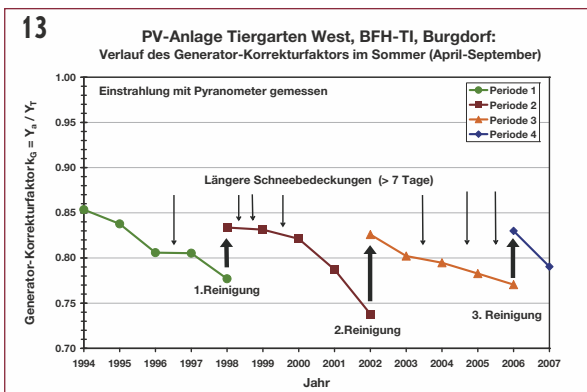
Bild 13 Gemessener Generator-Korrekturfaktor k_g bei der Teilanlage West der PV-Testanlage der BFH Burgdorf mit Angabe der Reinigungen (Strahlungsmessung mit Pyranometer). Die Anlage hat gerahmte Siemens M55-Module mit \beta = 30^\circ (horizontal liegend), liegt nahe bei einer Bahnlinie und neigt somit zu relativ starker Verschmutzung [8]. Der relativ tiefe Wert des Anfangswerts von k_g ist teilweise auf die gegenüber einer normalen PV-Anlage etwas höheren DC-Verluste der Testanlage zurückzuführen.
