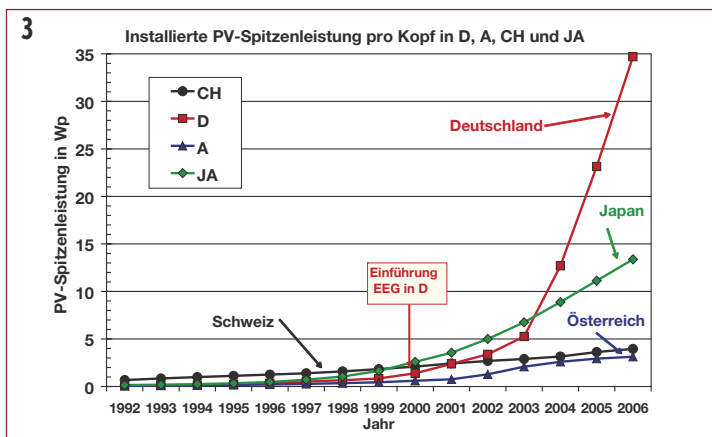
Bild 3 In Deutschland, Österreich, der Schweiz und Japan jeweils per Ende Jahr installierte totale PV-Spitzenleistung pro Kopf der Bevölkerung in den Jahren 1992 bis 2006 im Vergleich (Grafik aus [1], aufdatiert mit neuesten Werten aus [2]).
